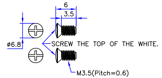
SCREW(2PCS)
