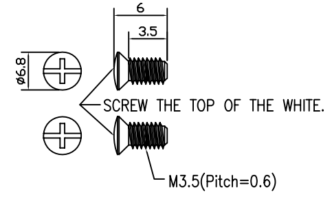
SCREW(2PCS)
