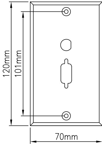
HDB15+3.5FT FACE PLATE(P/N:JPFP-HD15F-35F)
