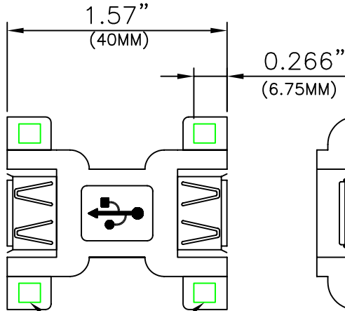
P2 USB A/F
