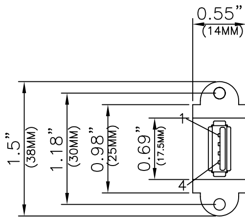
P1 USB A/F
