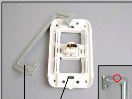
はさみ金具 取付枠部
