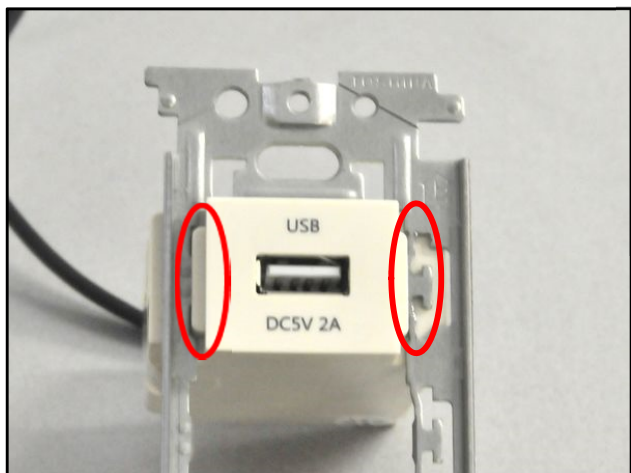
図1 N-USB0241を東芝製NDG4301に取り付けた例
