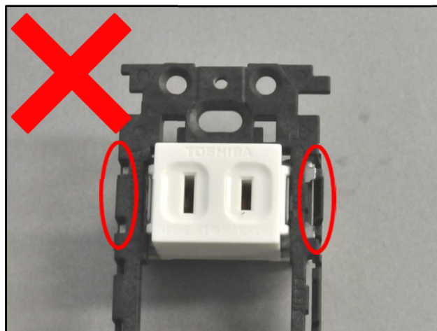
図2 東芝製絶縁枠NDG4302の保持例 赤丸部分を使用して保持します。
