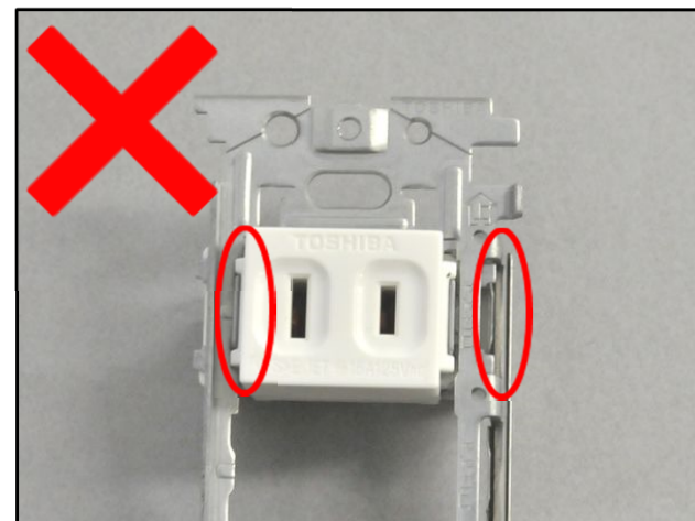
図3 東芝製ワンタッチ金属枠NDG4332の保持例 赤丸部分を使用して保持します。
