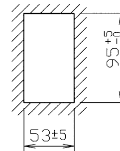
※壁の穴あけ寸法
