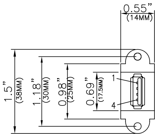
P1 USB A/F
