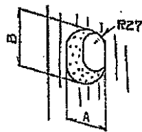
取付穴寸法
