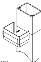
取付例： ダクトを突当てて接続し、継ぎ目にジョイントカバーを取付ける。
