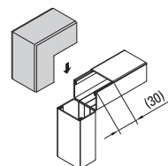
突当て接続時施工例
