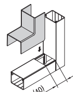
突当て接続時施工例2
