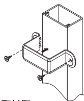
取付例： ダクトの上から固定バンドで固定する。
