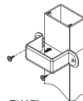
取付例： ダクトを突当てて接続し、継ぎ目に固定バンドを取付ける。
