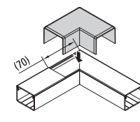
45°カット接続時施工例
