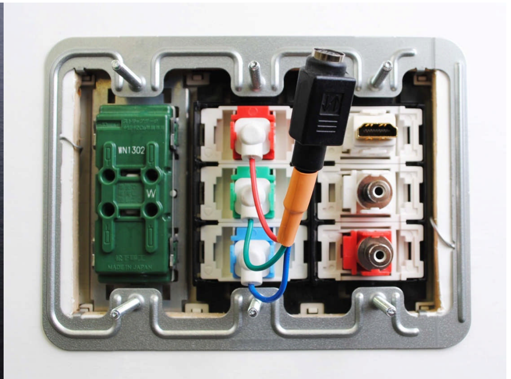
スナップイン中継コネクタの取付例 (裏面)
